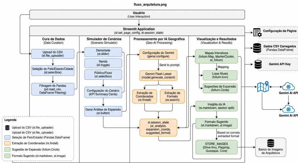
Figura 1 – Arquitetura Lógica e Fluxo de Dados do Sistema.
