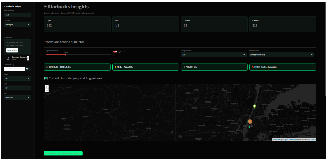
Figura 2 – Interface visual do sistema para análise de expansão comercial.
